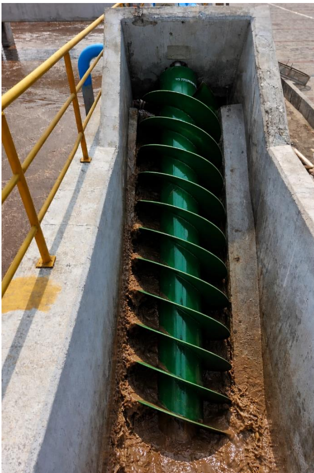
پمپ اسکرو ارشمیدسی تصفیه خانه فاضلاب اکباتان تهران
